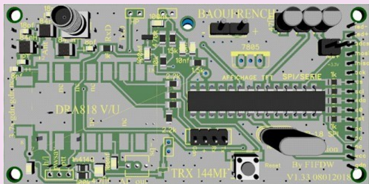
Circuits imprimés
