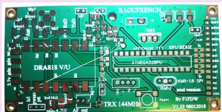
Circuits imprimés
