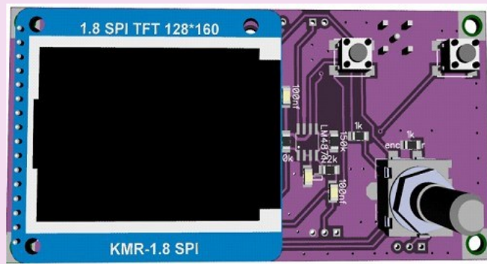
Circuits imprimés
