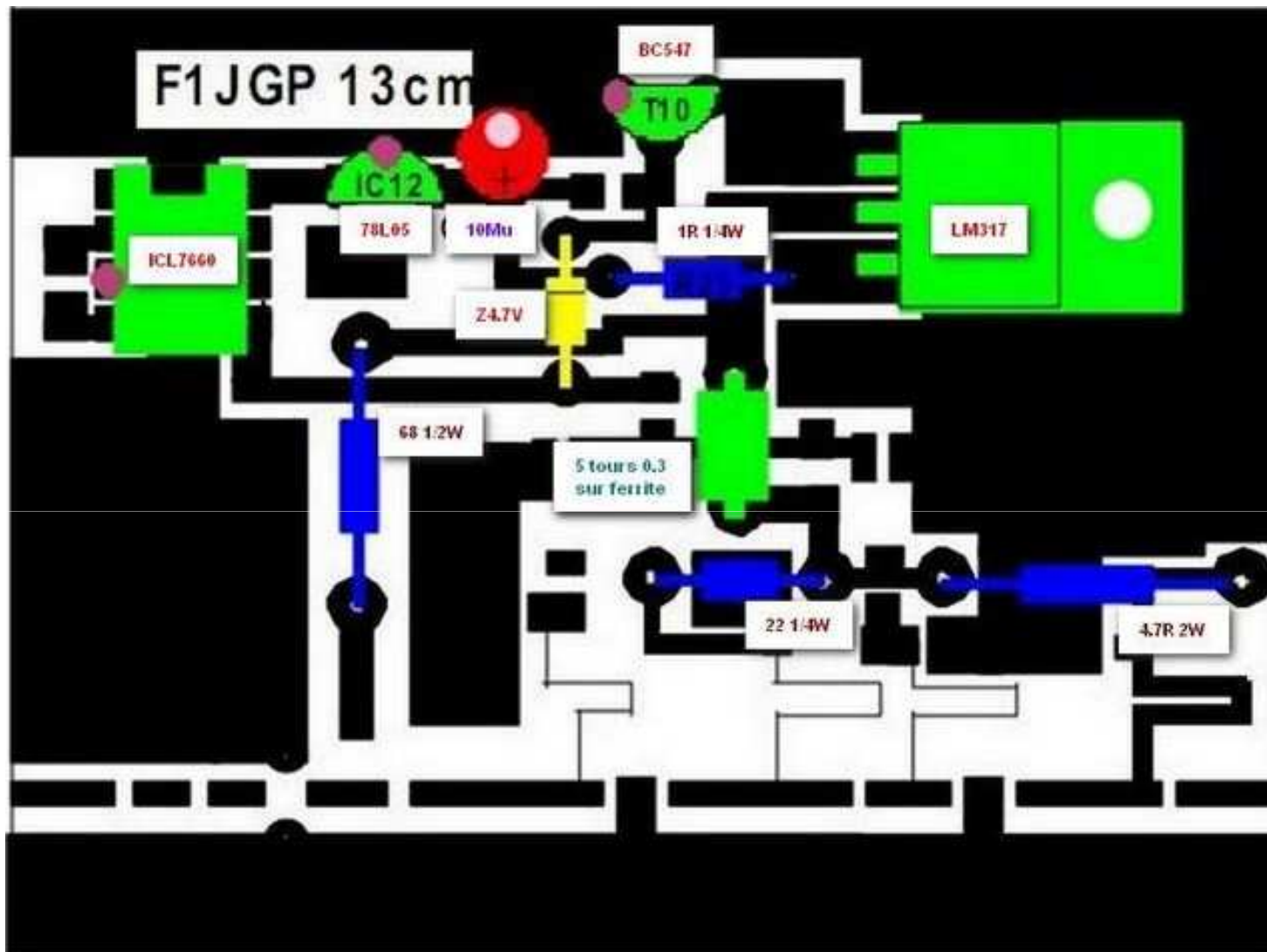
Circuit imprimé côté face RF (donc vu en transparence)
