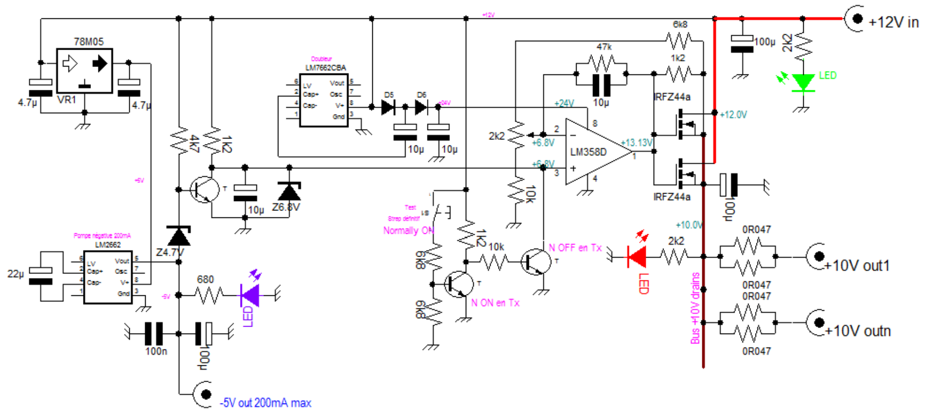
Alimentation originelle -5V et +10V de puissance F10PA F5DQK 1/2017
